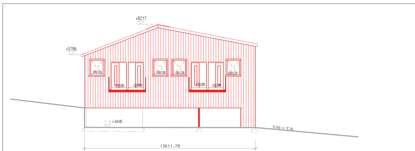
Façade sud-est / Südöstliche Fassade
