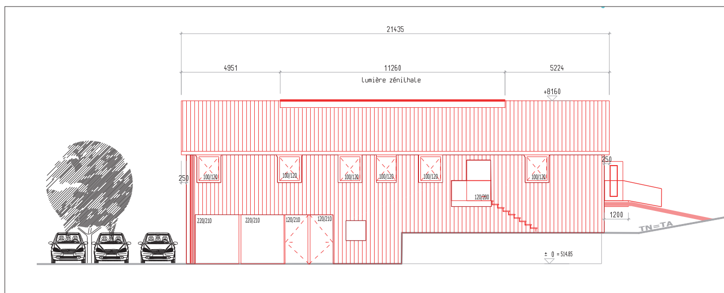
Façade sud-ouest / Südwestliche Fassade
