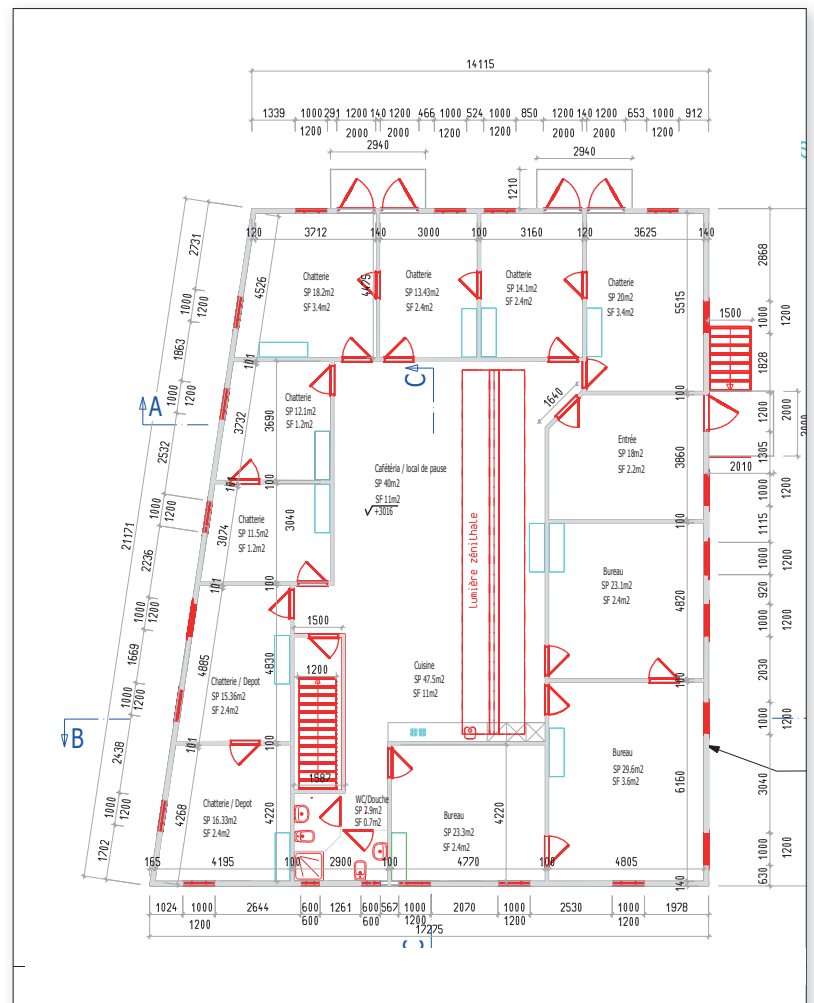
Premier étage / Erster Stock
