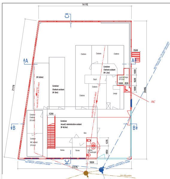
Rez-de-chaussée / Erdgeschoss
